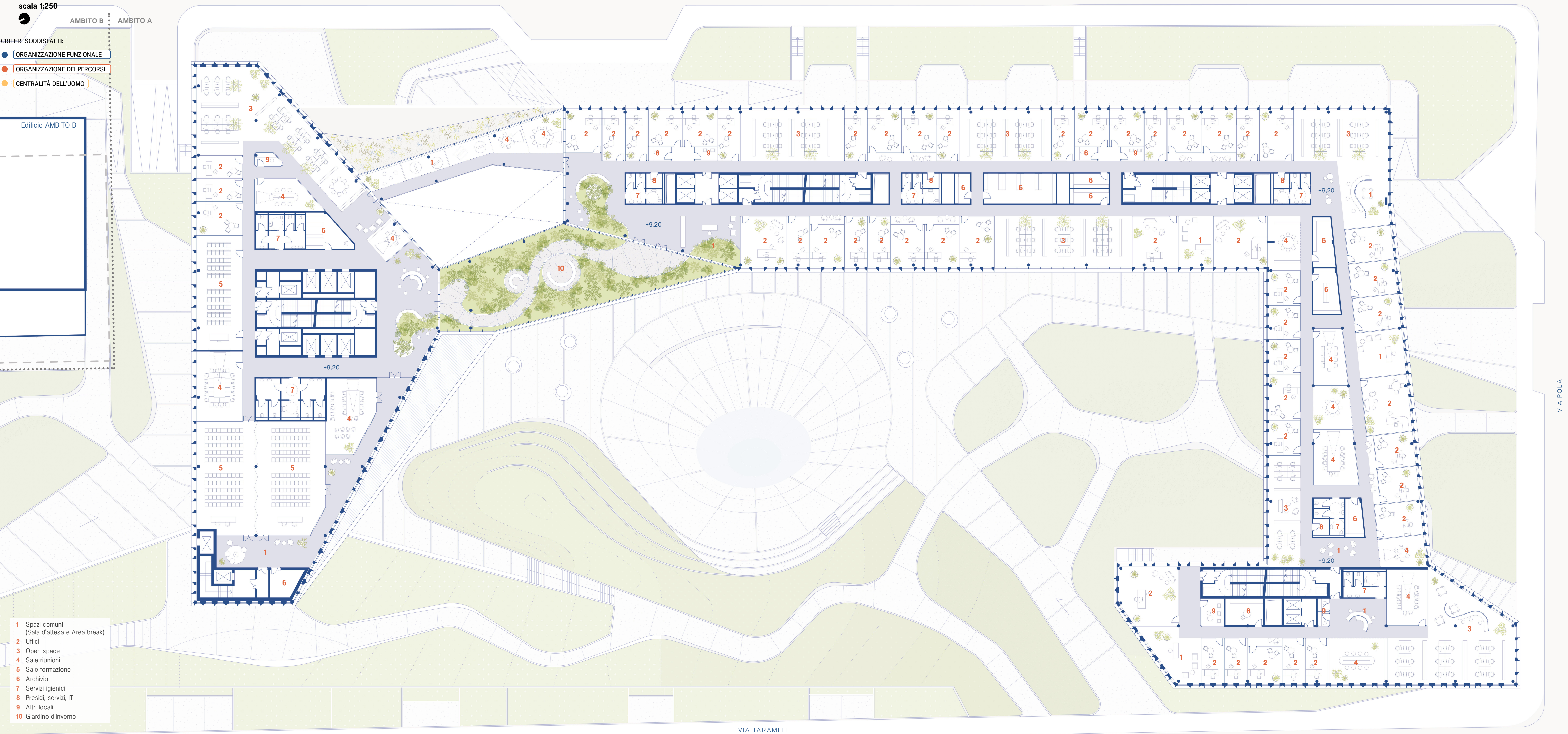
4.4 Pianta piano Primo
